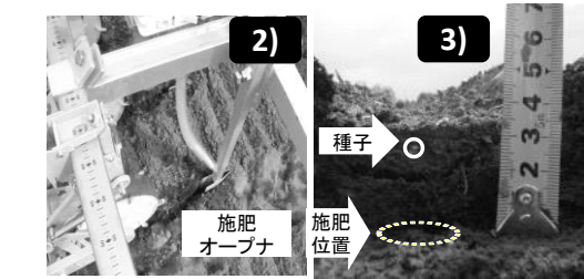
図 1 1) 施肥装置と播種機の模式図、2) 試験 に用いたオープナ(試作機)および、3) 覆土され た種子と肥料
