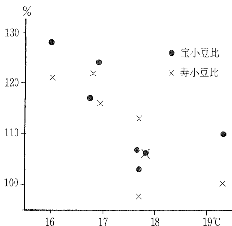
図2 6月～9月の平均気温と「エリモショウズ」の収量比 (1977～1983)
