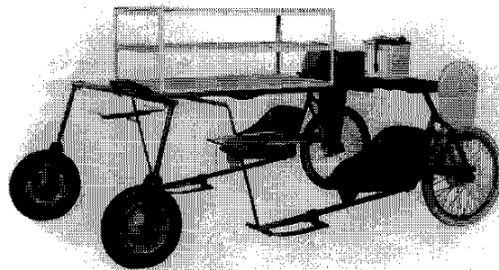
斜 視 図
