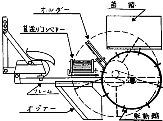
第41図 トランスplanter略図
