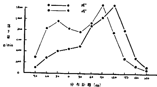
第51図 散布高さと分布
