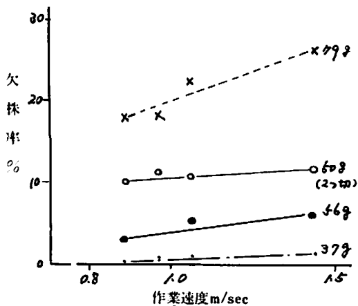
第36図 馬鈴薯重量別作業速度と欠播率の関係
