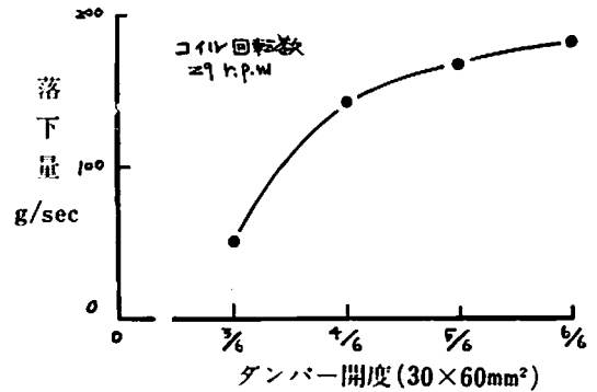
第27図 コイル式B型のダンパー開度と落下量の関係
