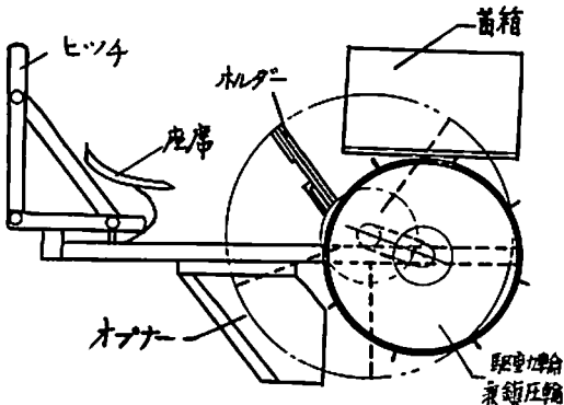
第40図 トランスプランター略図
