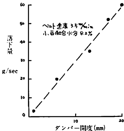
第30図 ダンパー開度と落下量の関係
