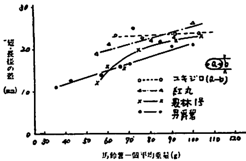
第24図 馬鈴薯平均重量と短・長径差の関係
