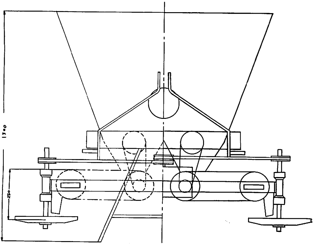
第 43 図 肥料散布機概略図 a
