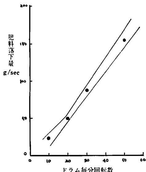
第21図 トラム回転数と落下量の関係
