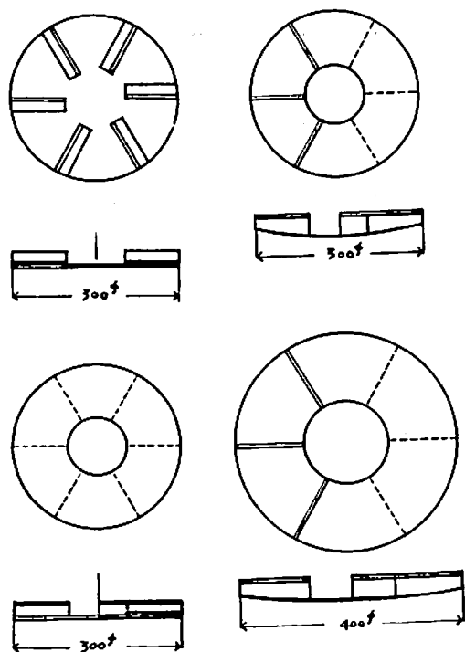
第47図 散布板形状
