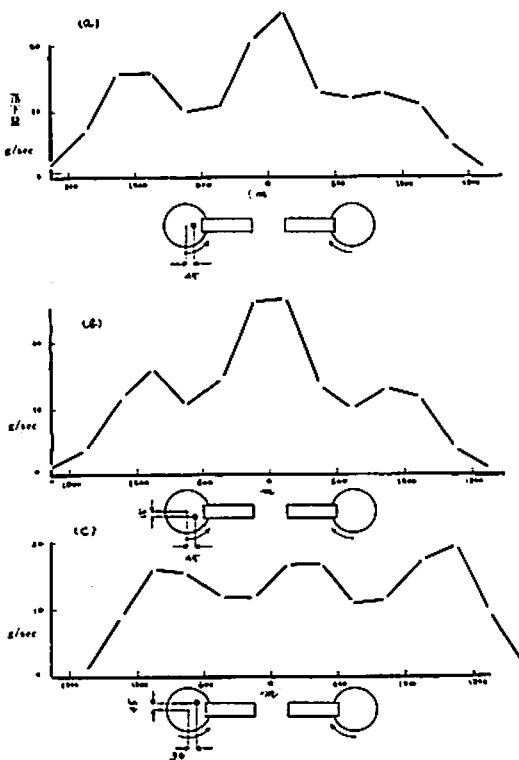
第54図 肥料落下着板位置 (石灰)
