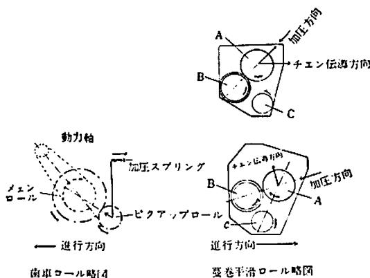
第 109 図 各試作機のロール関係位置
