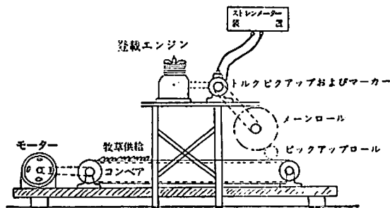
第110図 室内試験実験装置略図
