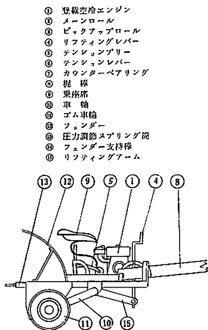
側面略図
