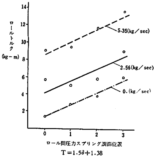
第113図 ロール間加圧とトルク変化
