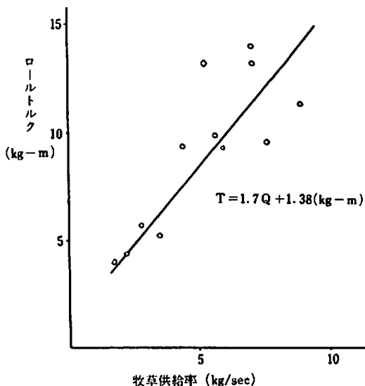
第112図 メインロール・トルクと牧草供給率の関係
