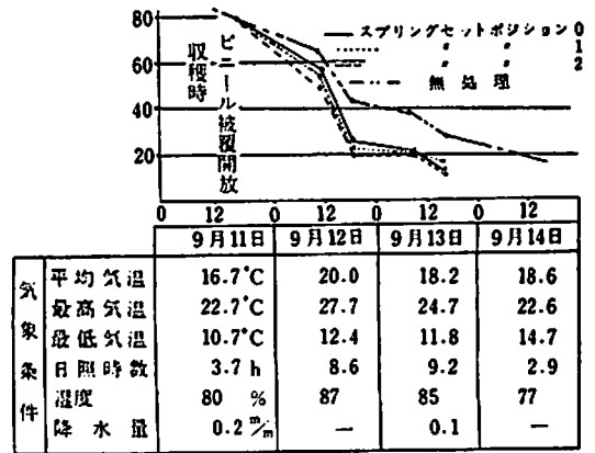
第119図 室内実験における牧草水分乾減状況 (ロール間圧力との関係)
