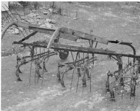
3. ウィダーカルチベーター (供試機) 〈53頁参照〉
