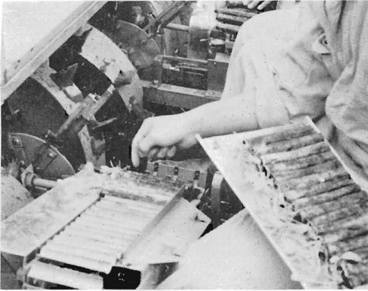
1. てん菜半自動苗送り装置 〈38頁参照〉
