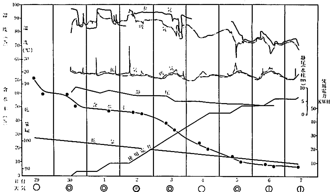
第10図 予乾、細断赤クロバーを供した乾燥実験の経過 (実験4)
