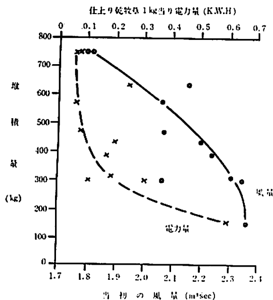
第16図 材料の堆積量と乾燥効果
