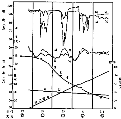
第7図 非予乾赤クロパーを供した乾燥 実験の経過 (実験1)
