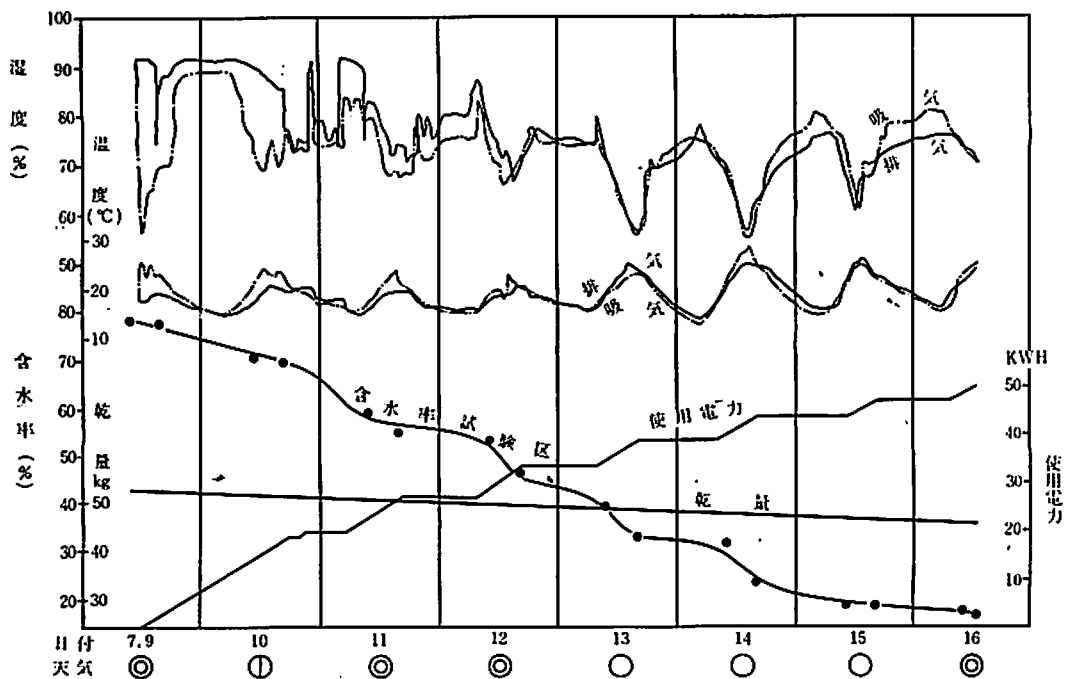
第 9 図 非子乾, 非細断赤クロバーを供した乾燥実験の経過 (実験 3)
