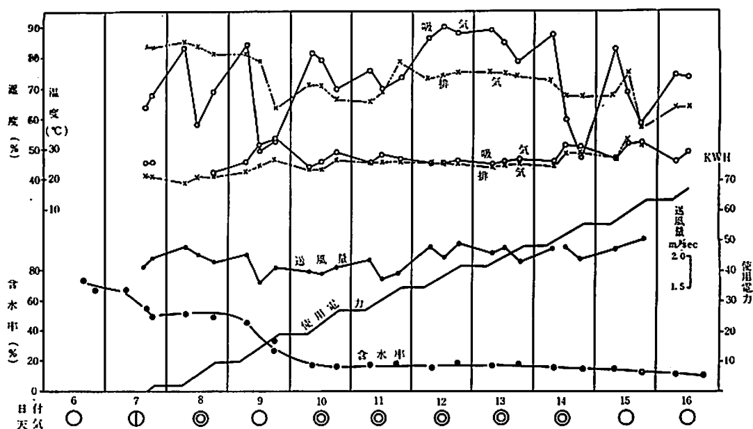
第12図 予乾、細断赤クロバを供した乾燥実験の経過 (実験6)
