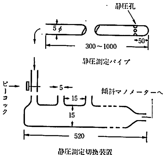
第5図 静圧測定装置
