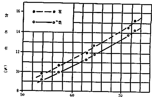
図 1 レンゲの平衡水分
