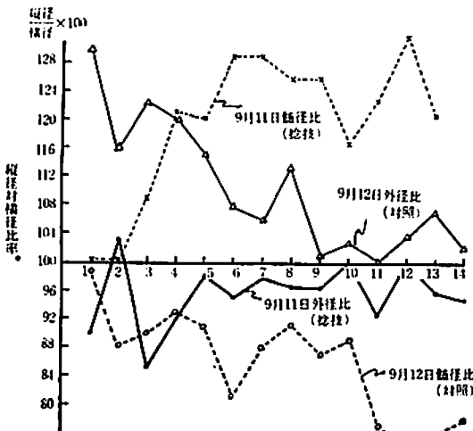
第16図 90度振廻による枝形と髓形との関係 (注) 品種「デラウエア」
