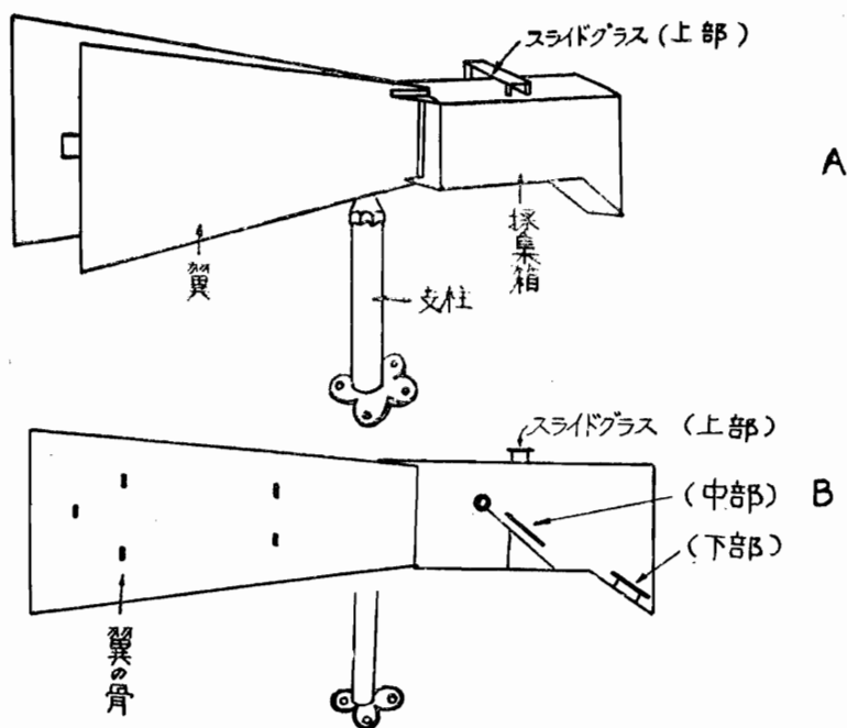
第1圖 胞子採集器
