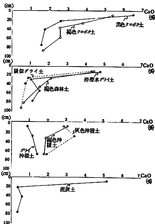
図-26 土壌亜型別 CaO 含量の比較
