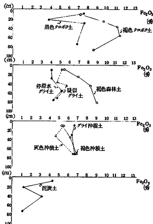
図-24 土壌亜型別 \text{Fe}_2\text{O}_3 含量の比較
