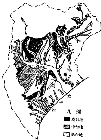
図-6 十勝平野の概括的地形区分図
