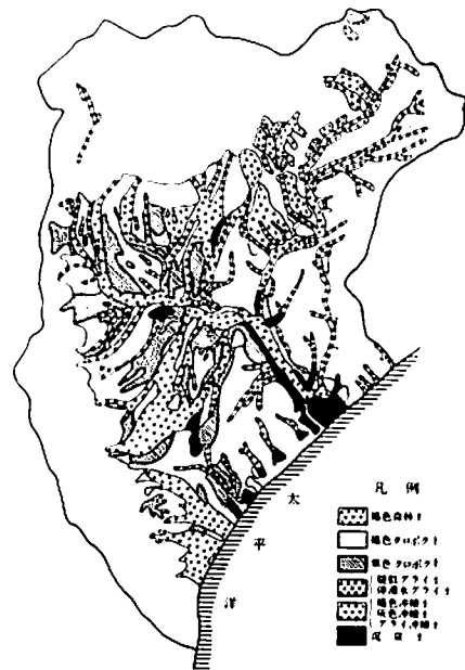
図-20 十勝平野の土壌分類図Ⅰ(土壌型)
