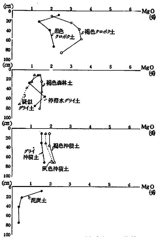
図-27 土壌亜型別 MgO 含量の比較
