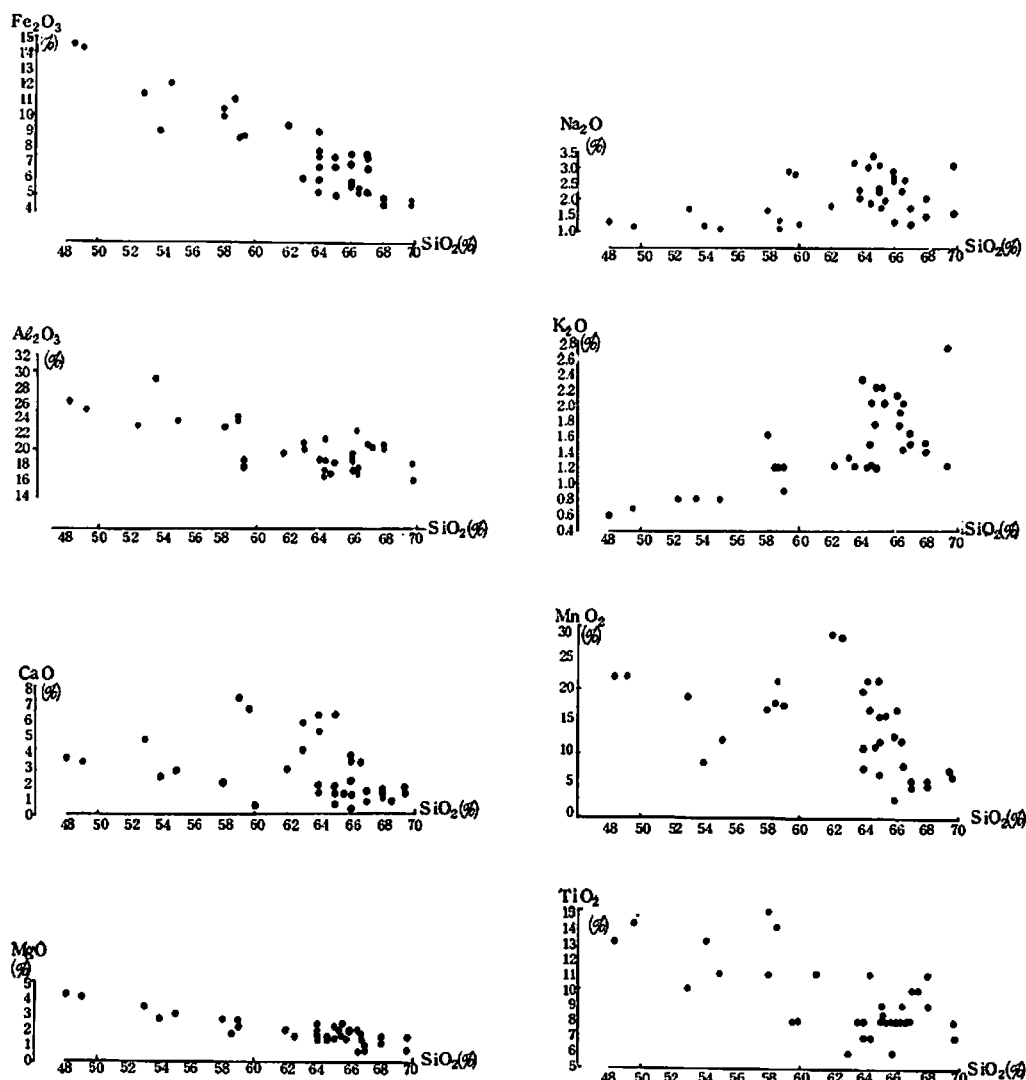
図-33 土壌の \text{SiO}_2 含量と化学成分との関係
