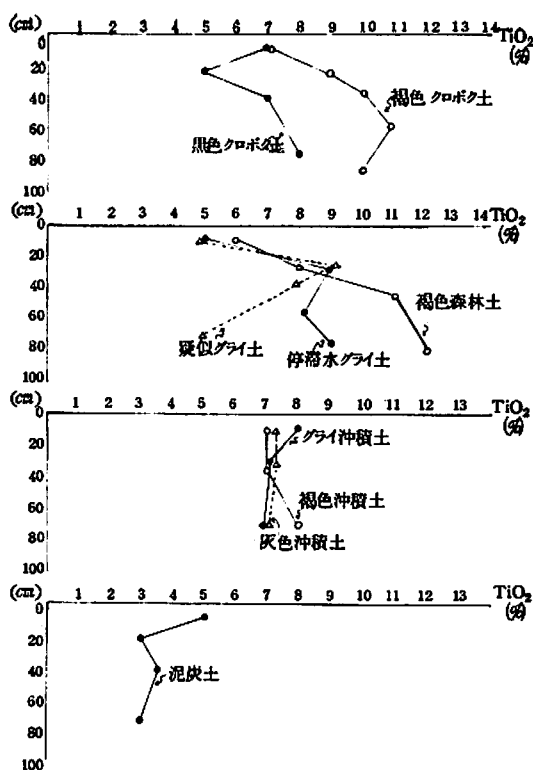
図-31 土壌垂直型別 \text{TiO}_2 含量の比較
