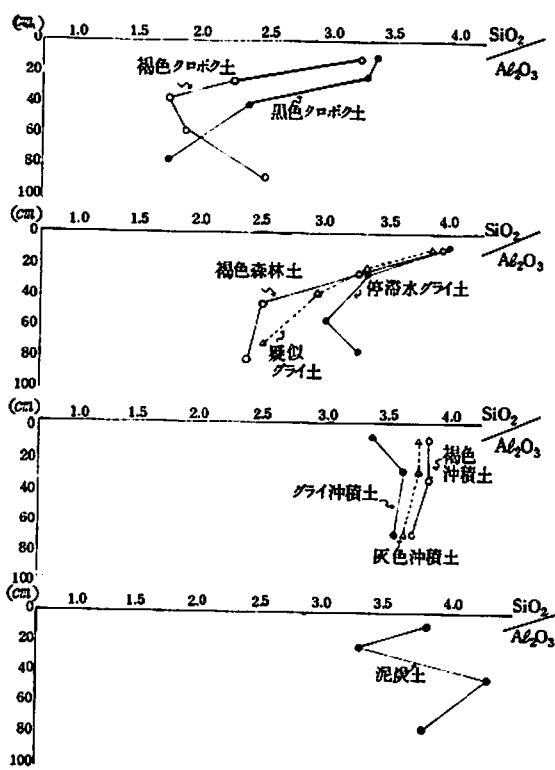
図-32 土壌垂直型別 \text{SiO}_2 / \text{Al}_2\text{O}_3 含量の比較
