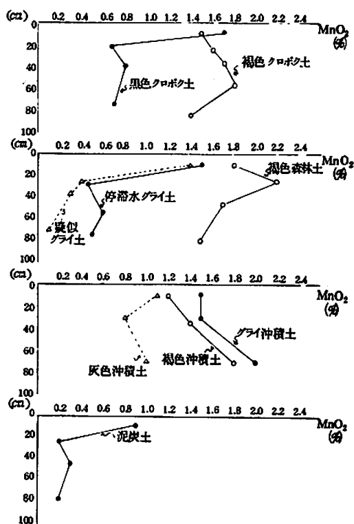
図-30 土壌垂直型別 \text{MnO}_2 含量の比較
