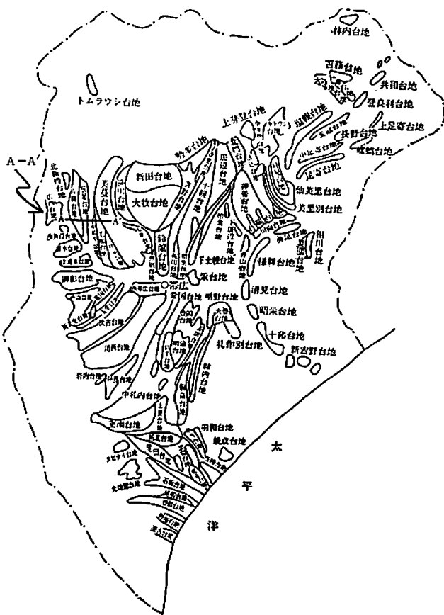
図-1. 十勝の台地区分図
