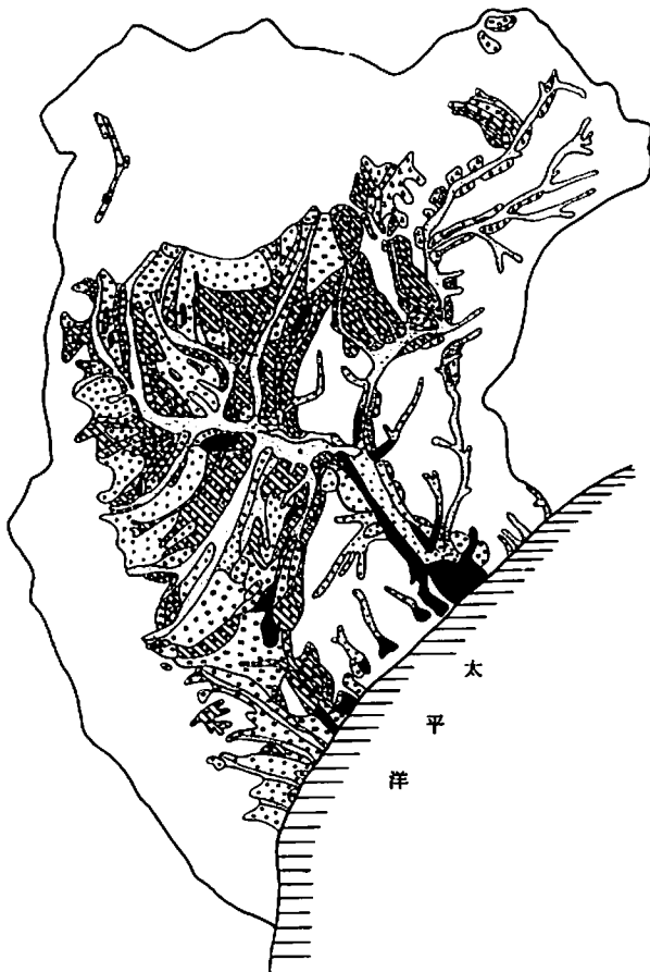
図-21 十勝平野の土壌分類図Ⅱ(土壌属)
