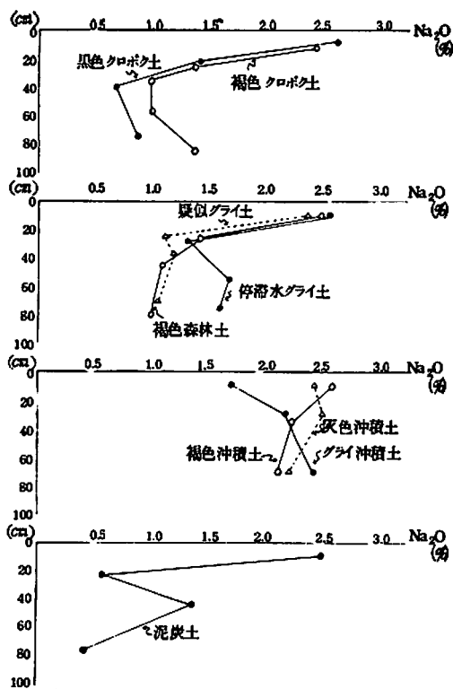
図-29 土壌垂直型別 \text{Na}_2\text{O} 含量の比較
