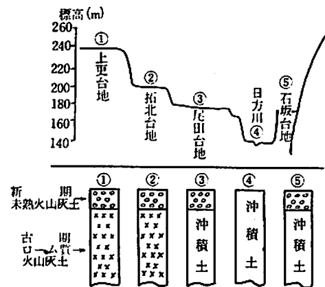
図-16 区分した火山灰の堆積関係 その2 (南部)
