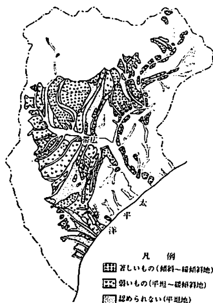
図-3 台地の侵食の状況
