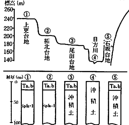
図-10 火山灰と地形面との堆積関係 その2 (南部)
