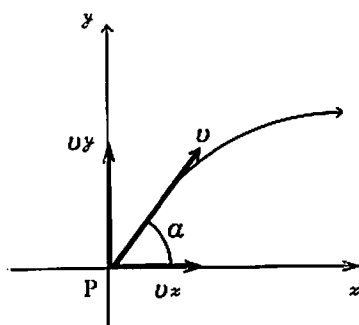
図 59. 石礫の放出軌跡
