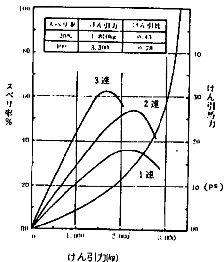
図86 80PS級四駆型トラクタけん引性能
