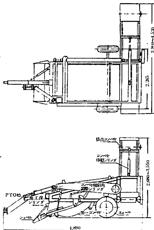
図 63 Y S 1,400 型 ( ストーンピッカ )
