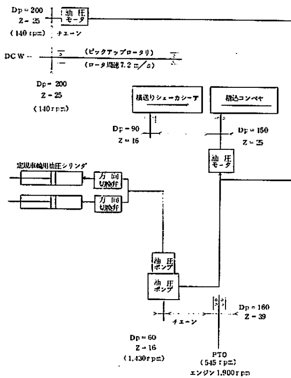
図 5 3 動力伝達系統図
