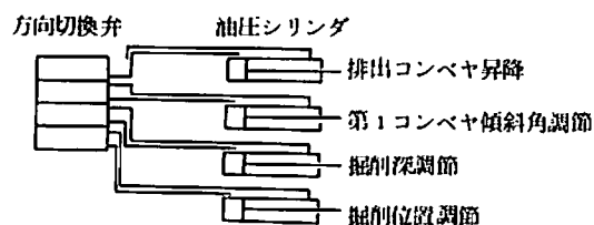
図 65 油圧系統図
