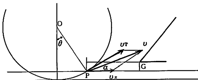
図 60. タインの作用図
