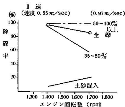
図 8 1 回転数別除礫率
