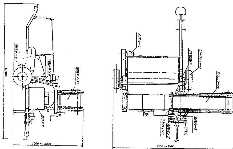
図 5 2 フェーズ D - 2000 型 ( ストーンコレクタ )
