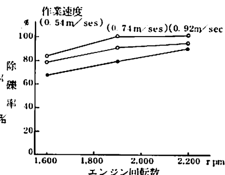
図 56. 回転数と除礫率
