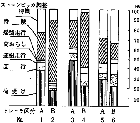
図 7 6 トレーラの工程別時間割合
