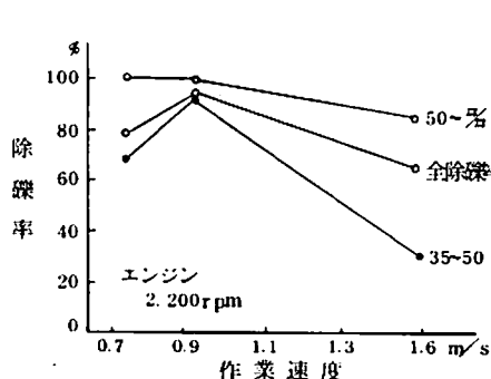
図 55. 作業速度と除礫率
