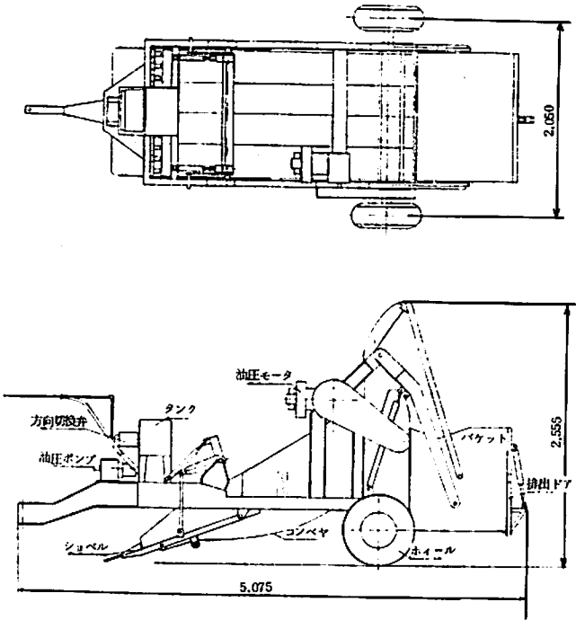
図 68 ST 1,500 型 (ストーンピッカ)
