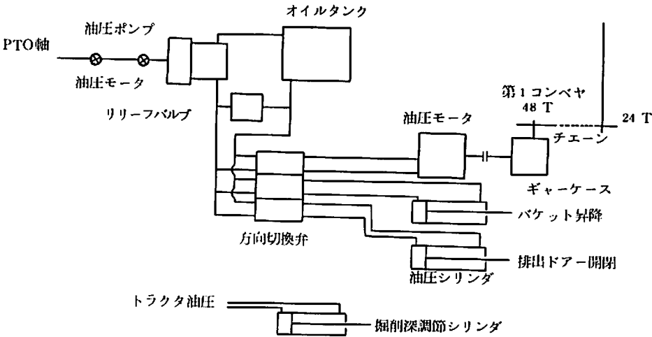
図 68 ST 1,500 型 (ストーンピッカ)
