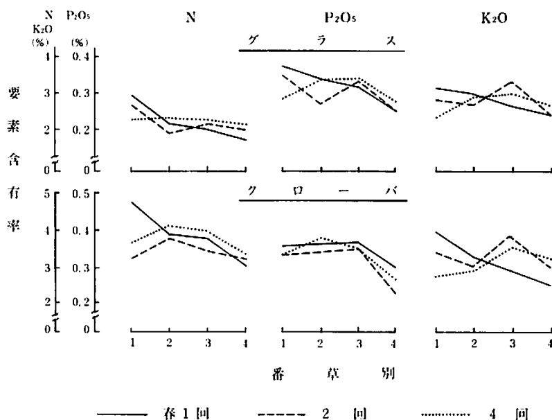
第30図 各刈取りごとのN, P_2O_5 , K_2O 含有率(5種混播, 1年目)
