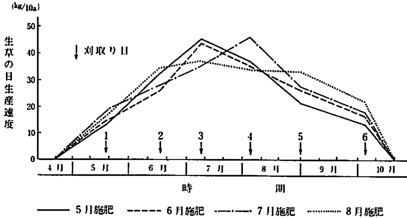
第37図 A試験における生草の日生産速度の推移(2年目)
