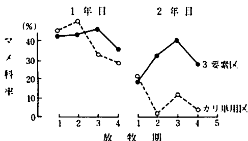
第34図 マメ科率の推移
