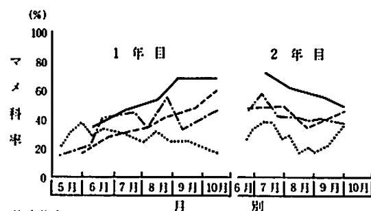
第33図 入牧時の草丈とマメ科率の推移
