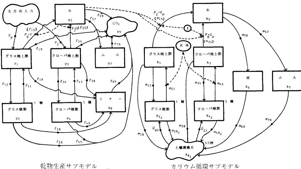
図37 コンパートメントモデル
