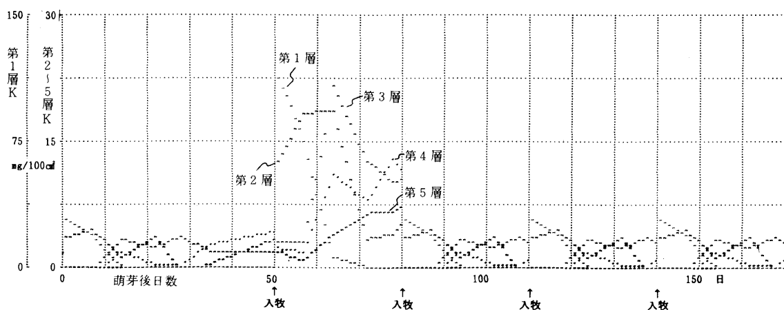
図38 土層別、土壤溶液 K の推移 (シミュレーション, カリウム循環サブモデルのインプット)
