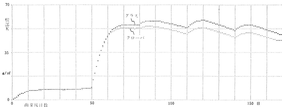
図41 牧草根部カリウム量の推移 (シミュレーション結果)
