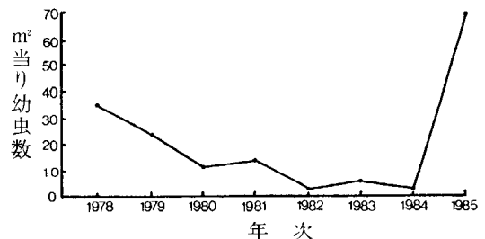
第2図 水田畦畔におけるヒメトビウンカ越冬後幼虫密度の変動
