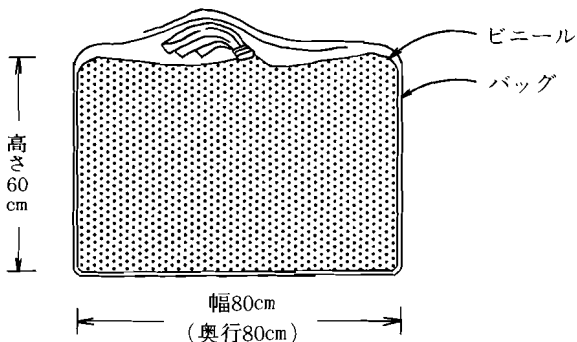
図37 脱水澱粉粕の貯蔵法
