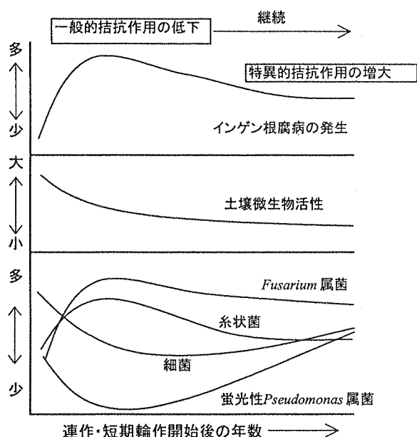
図VII-1 連作、短期輪作下のインゲン根腐病によぼす土壌微生物特性(模式図)
