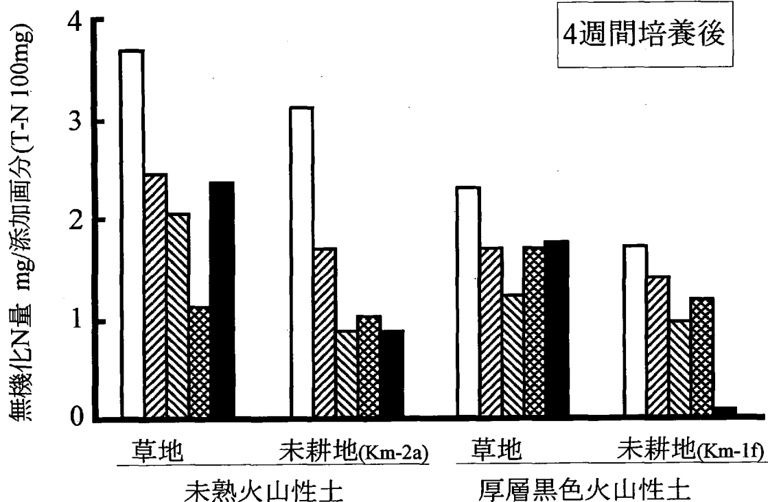
図4-9 添加した各画分(T-Nとして100mg相当量)からの無機化窒素量
