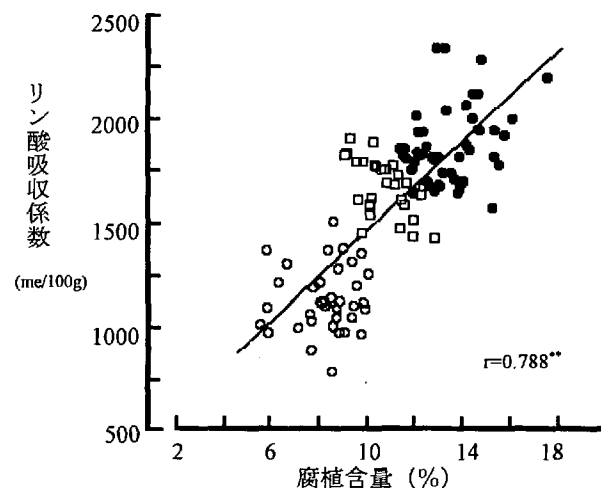
図3-14 土壌の腐植含量とリン酸吸収係数の関係
