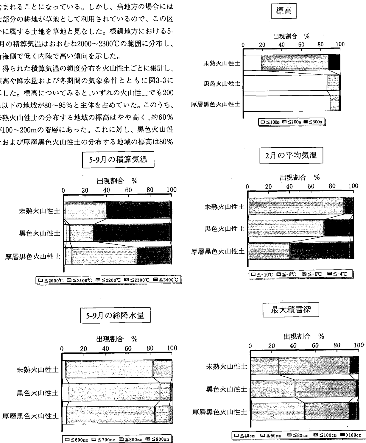
図3-3 根釧地方の主要火山性土における農耕地*の標高と平年の気象条件
