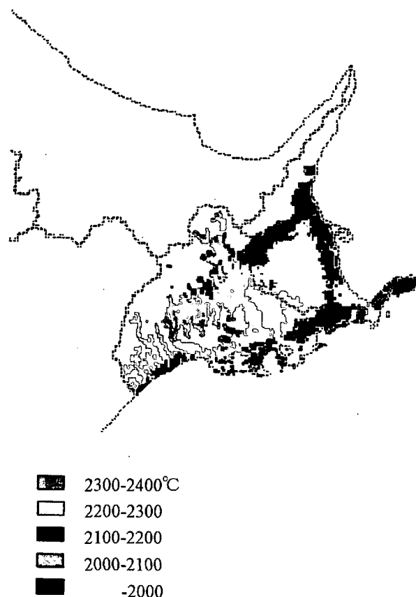
図3-2 根釧地方の農耕地*における5-9月の積算気温(平年値)
