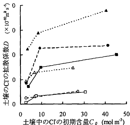
図3-18 土壤中のCl⁻の拡散係数に及ぼす
