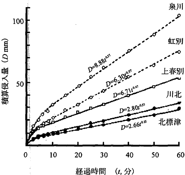
図3-10 水の積算侵入曲線
