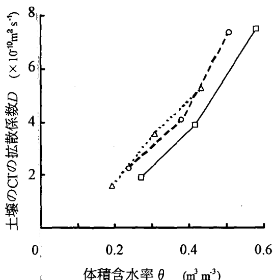
図3-17 土壤中のCl⁻の拡散係数に及ぼす
