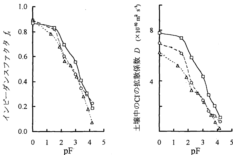
図3-20 pFとインピーダンスファクタおよび土壌中のCl - の拡散係数の関係
