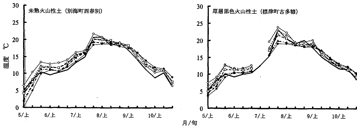
図4-7 未熟火山性土および厚層黒色火山性土の試験地における気温および地温の推移(1989年)
