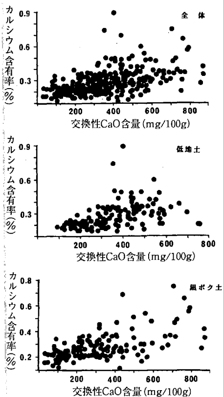
図Ⅲ-2 土壌別交換性石灰含量と牧草中のカルシウム含有率の関係
