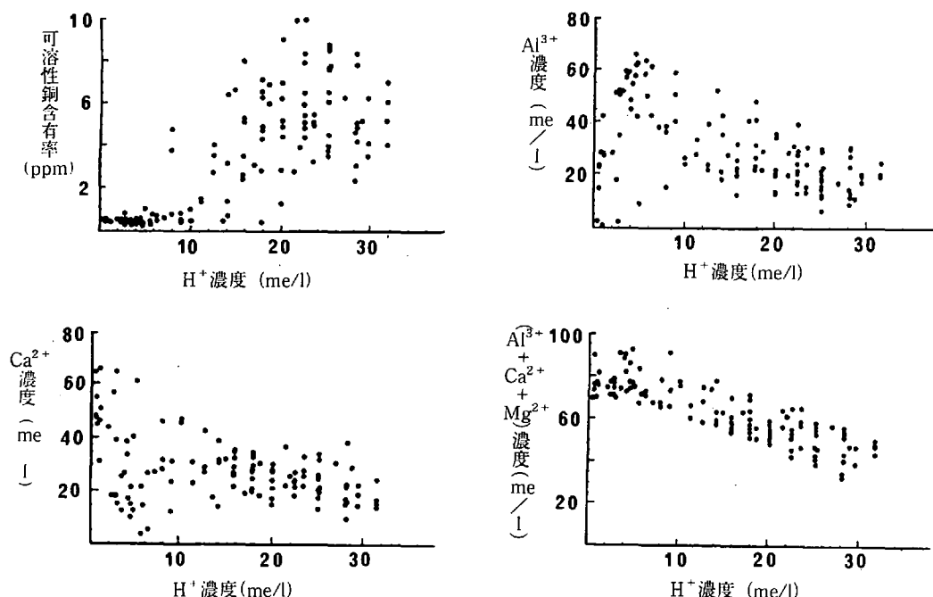
図Ⅱ-11 0.1N塩酸抽出液中の H^+ 濃度と可溶性銅含有率， 0.1N塩酸抽出中の Al^{3+} 、 Ca^{2+} の濃度および ( Al^{3+}+Ca^{2+}+Mg^{2+} )濃度との関係
