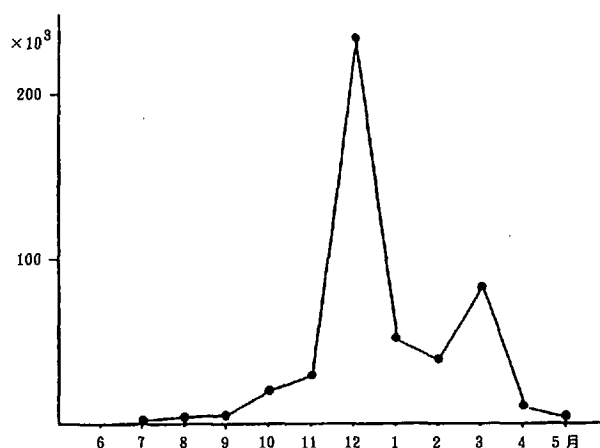
第13図 条斑病の多発生圃場における土壌中の病原菌数の推移
