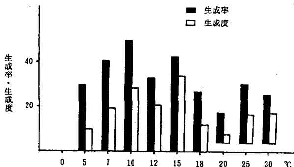
第1図 温度条件とコムギ条斑病菌スポロドキアの生成
