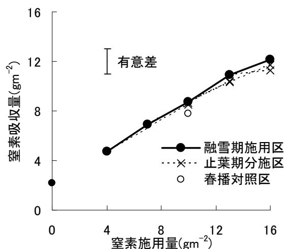
図2-2-3 窒素施用量と窒素吸収量との関係.
