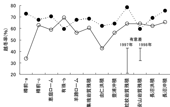
図3-2-1 越冬率の年次および土壌別の変動.
