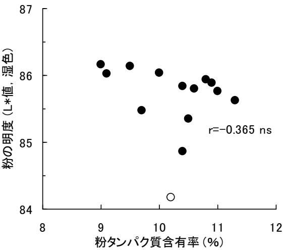
図 2-3-1 粉タンパク質含有率と粉の明度 (L*値) との関係 (3 カ年の平均値). ● 初冬播区, ○ 春播対照区. 相関係数は初冬播区の値 (標本数=13), nsは有意性なしを示す.
