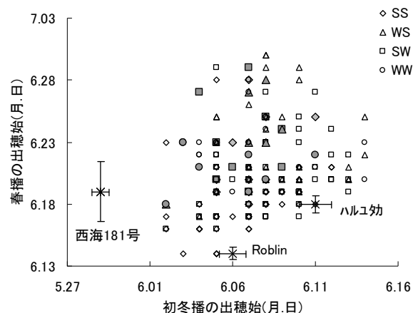
図 4-1-4 F 5 世代における初冬播栽培と春播栽培の出穂始の関係（2000 年）．
