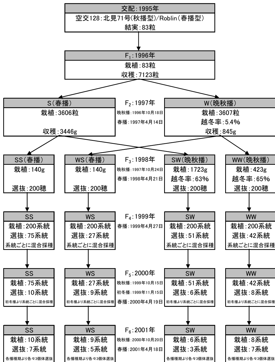
図 4-1-1 空交 128 の選抜経過.
