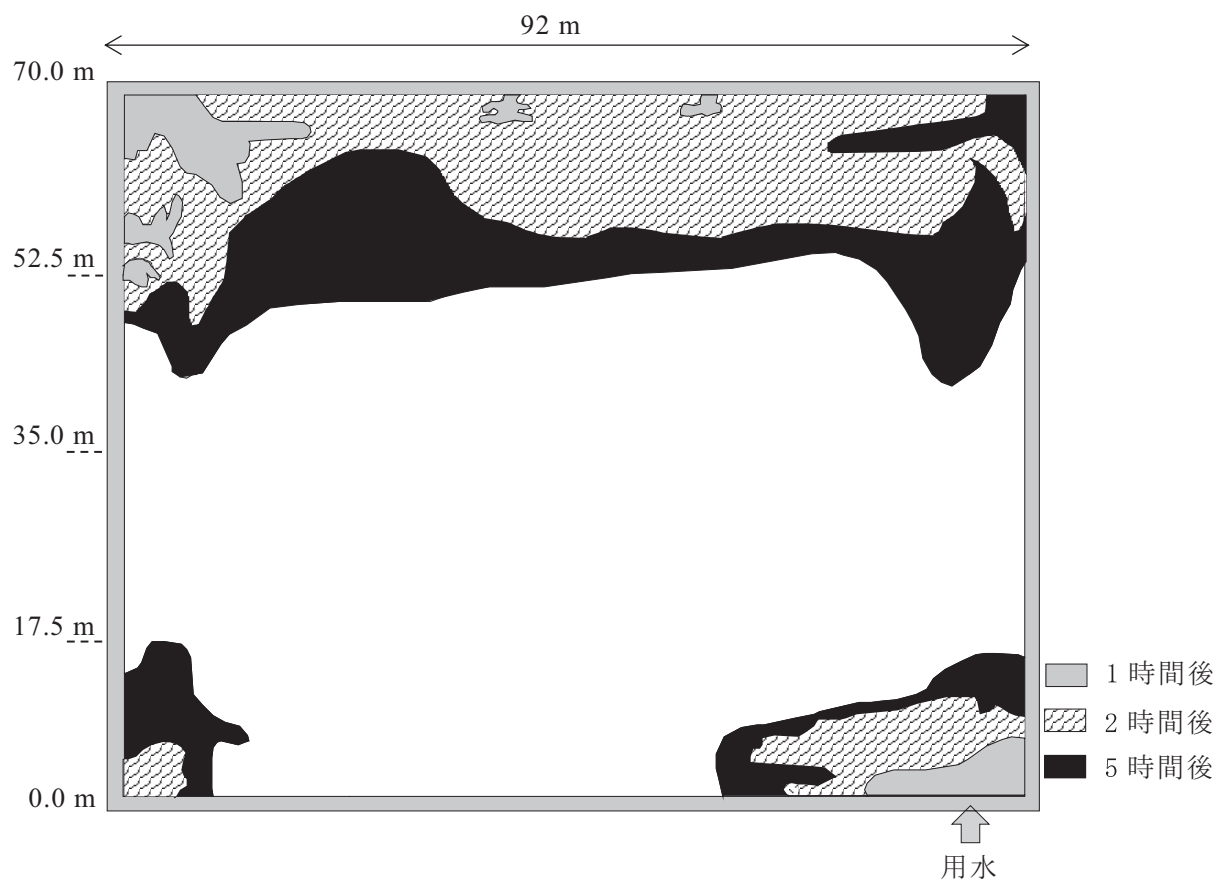
図 3-1-2 圃場内外周の溝に水を流した際の水足の広がり状況（調査圃場：C08）
