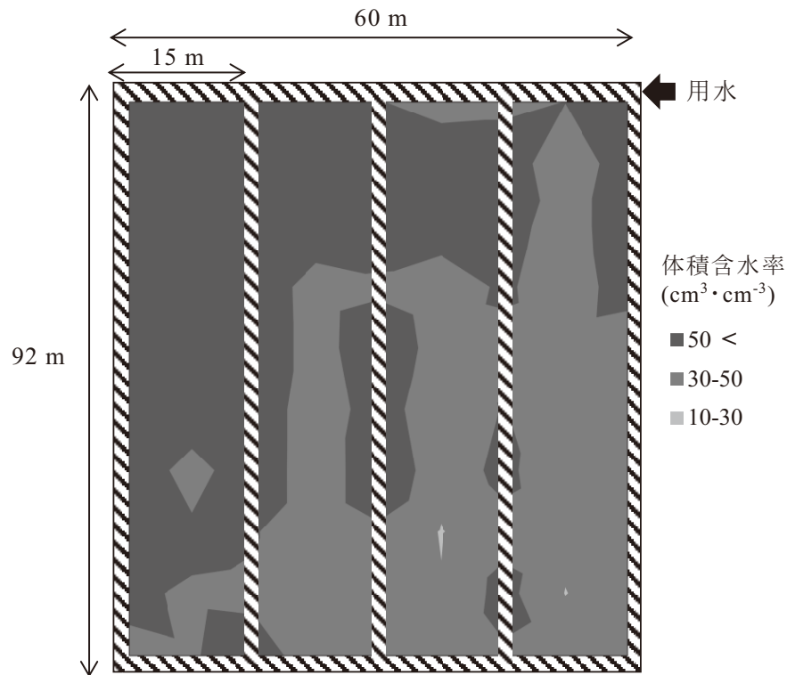
図 3-1-3 圃場内の外周ならびに長辺方向に 15m 間隔で溝を施工した圃場に灌漑した際の 9 時間後における体積含水率の分布
