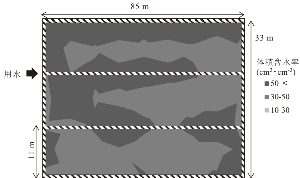
図 3-1-4 圃場内の外周ならびに長辺方向に 11m 間隔で溝を施工した圃場に灌漑した際の 8 時間後における体積含水率の分布
