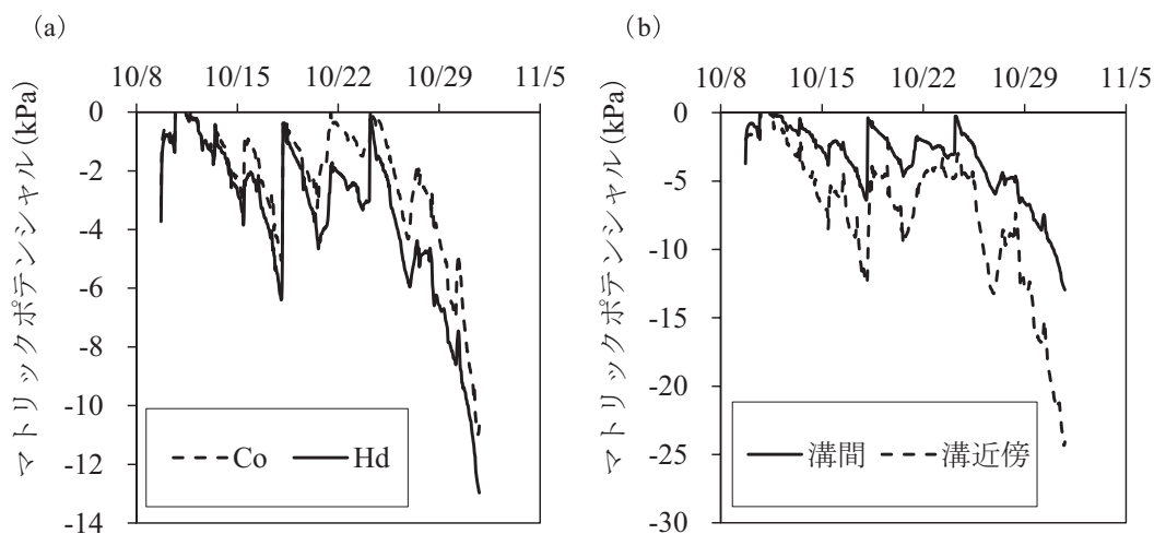
図 3-1-5 播種後から積雪前までの期間におけるハイブリッド水路施工区ならびに対照区の地表下 10cm 位置におけるマトリックポテンシャルの変動 (調査圃場: C09, 調査年: 2009, a: ハイブリッド水路施工区の溝間の値とハイブリッド水路未施工の対照区の値, b: ハイブリッド水路施工区内における溝間の値と溝近傍の値)
