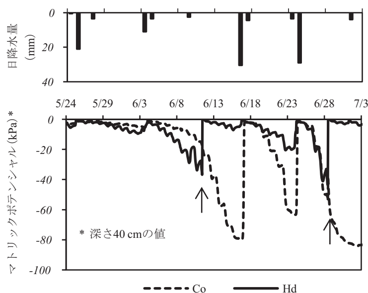
図 3-1-8 灌漑期間中に降雨を遮断したモデル試験におけるマトリックポテンシャルの推移 (調査圃場：C10-1，調査年：2010 年，)
