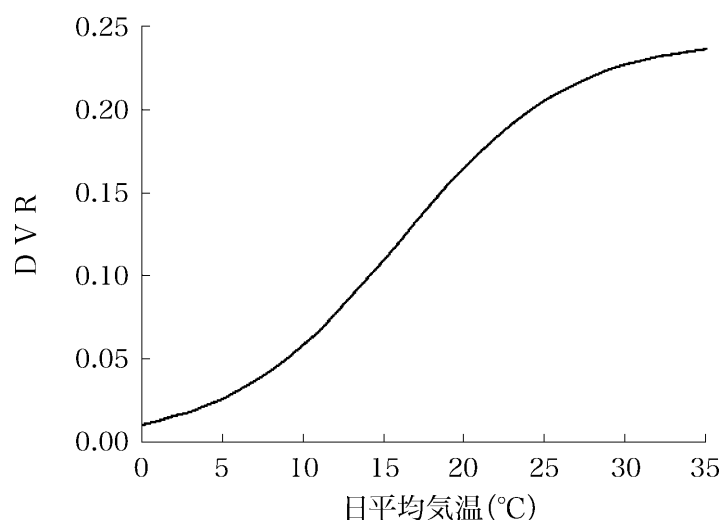
図3-5 日平均気温と播種から入水日までの1日当たり発育速度(DVR)の関係
