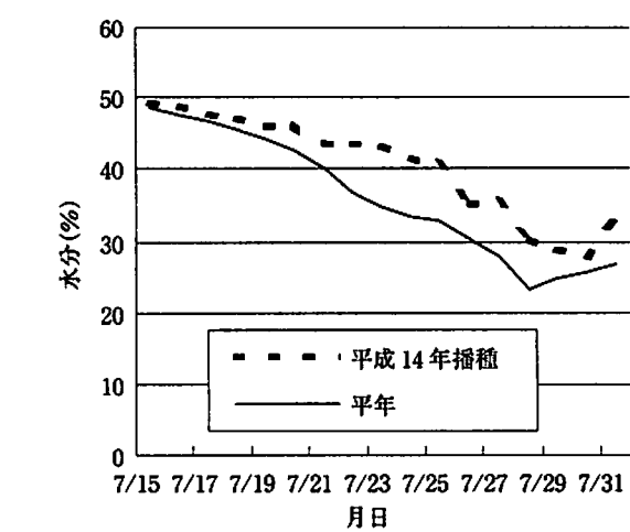
図Ⅲ-2-1-1 十勝農試における「ホクシン」の子実水分の推移 注）平年値は前 10 年の平均値。
