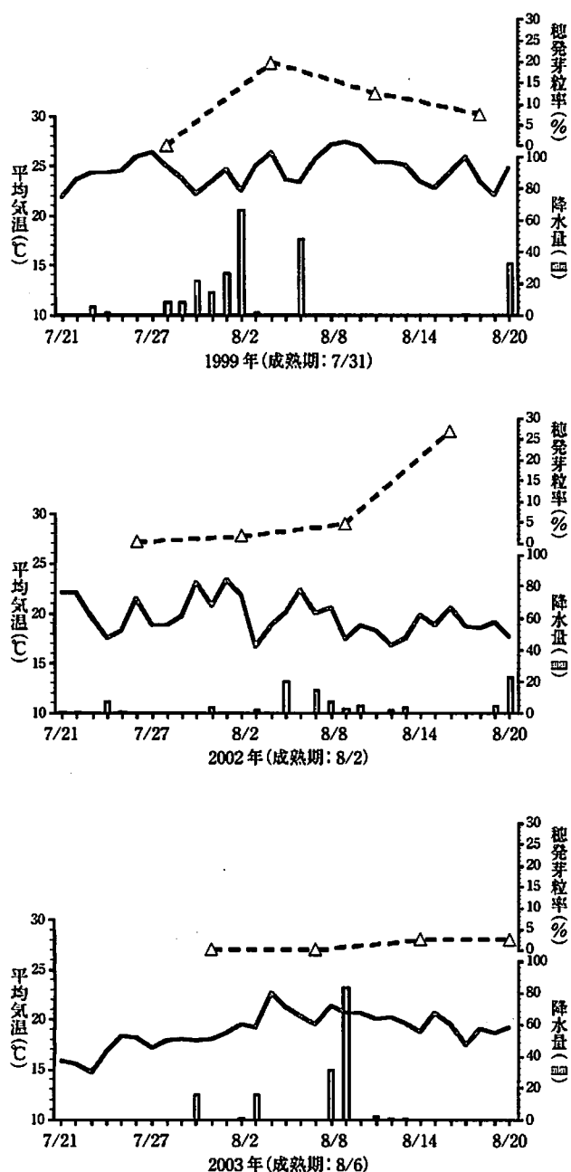
図III-2-1-8 成熟期前後の平均気温・降水量と穂発芽粒率の推移。品種「ハルユタカ」
