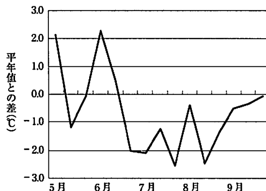
図Ⅲ-2-2-2 高収年(平成 14, 15 年平均値)における平均気温の推移
