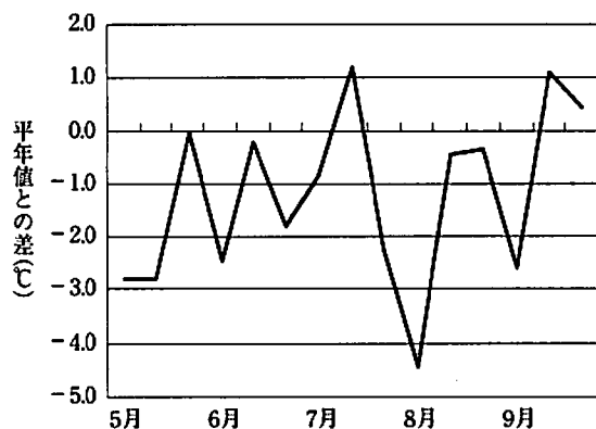
図Ⅲ-2-2-1 低収年(平成 5, 8 年の平均値)における平均気温の推移
