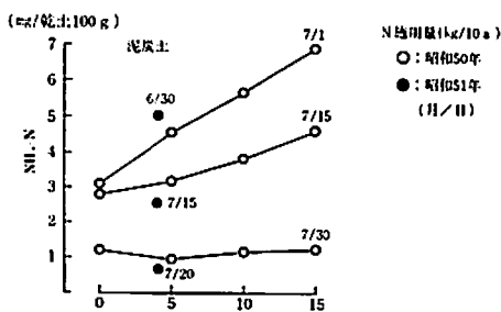
図Ⅳ-14 N施用量別の土壌中の \text{NH}_4\text{-N}
