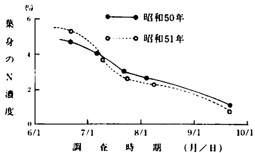
図IV-2 葉身のN濃度推移
