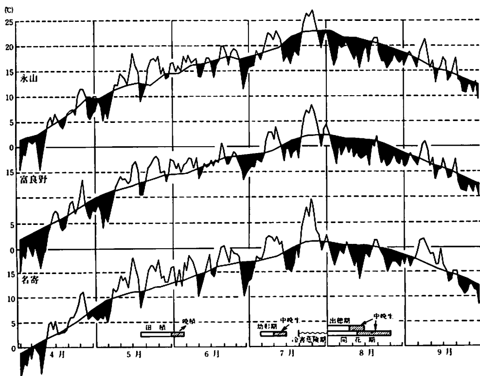
図Ⅱ-4 昭和51年の永山・富良野・名寄における気温の推移（日平均気温）
