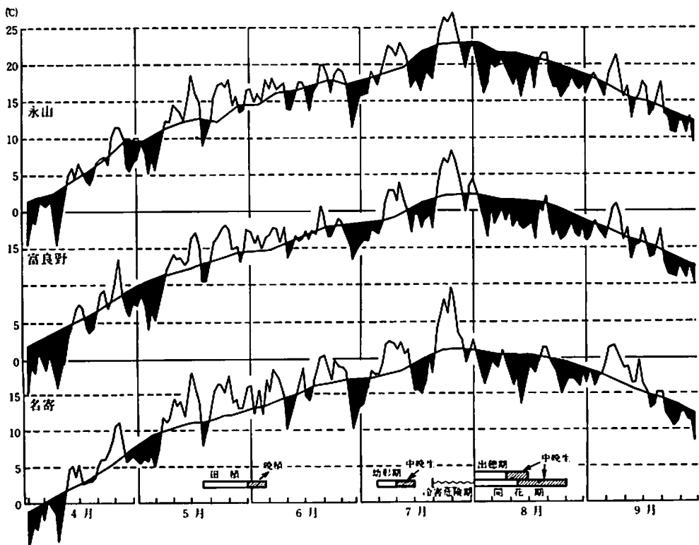
図Ⅱ－４ 昭和51年の永山・富良野・名寄における気温の推移（日平均気温）
