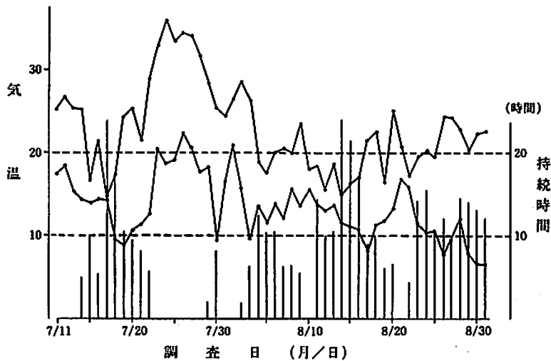
図II-2 7・8月の日別最高最低気温と15℃以下持続時間
