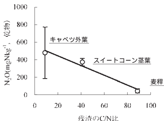
図4 残渣のC/N比と残渣の乾物1kg当たりから発生した N_2O との関係(試験3)
