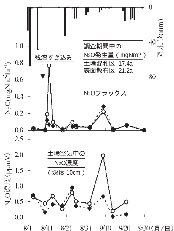
図5 キャベツ外葉残渣のすき込み方法の違いが N_2O フラックスおよび土壌空气中的 N_2O 濃度に及ぼす影響(試験4)
