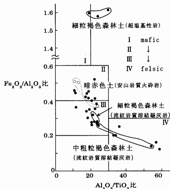
図2 Al_2O_3/TiO_2 比と Fe_2O_3/Al_2O_3 比の関係
