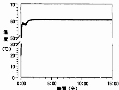
図1 60°C15分処理における粃直近温度の推移 注) もみ温度19.4°C 2kg2袋で処理した。
