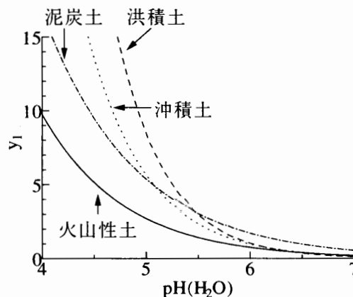
図3 堆積様式別にみたpHと y_1 の関係 (畑・草地)
