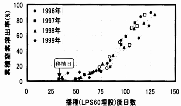
第1図 被覆尿素肥料(LPS60)からの累積窒素溶出率の推移 ○；幼穂形成期 □；出穂期
