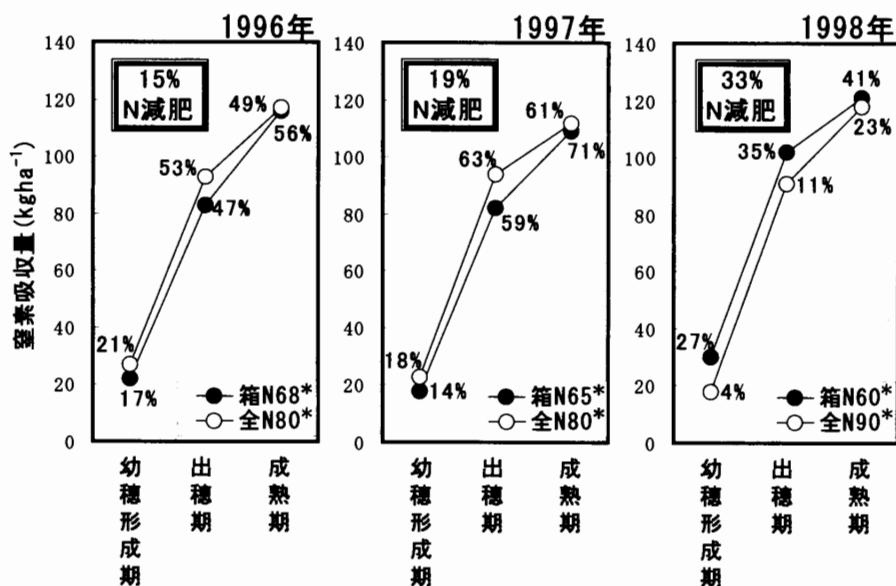
第2図 全量育苗箱施肥区の窒素吸収量の推移 (添え数字は施肥窒素利用率)
