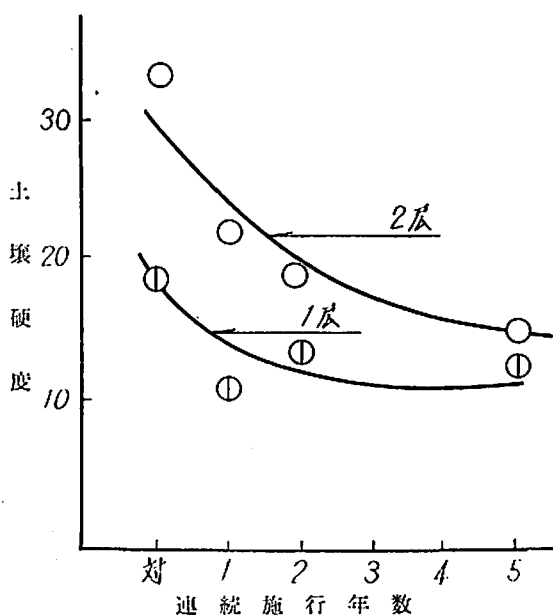
第5図 土壌硬度
