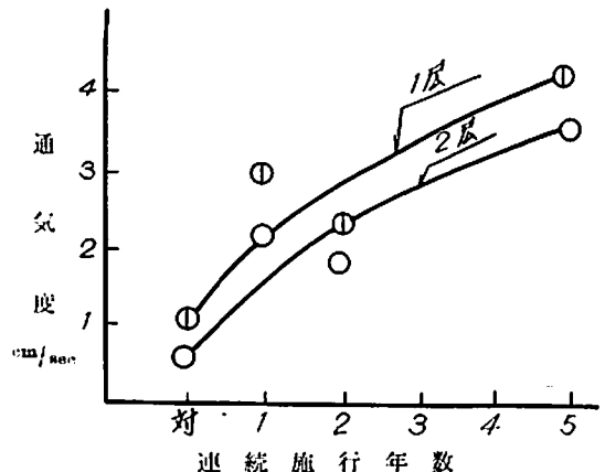
第2図 通気度
