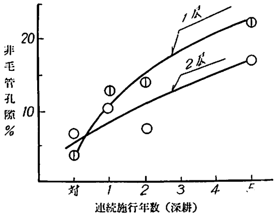
第1図 非毛管孔隙
