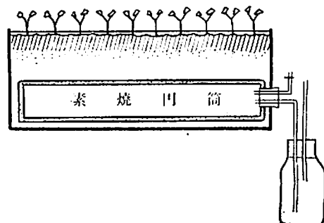
第9図 自給灌水用吸水量測定装置
