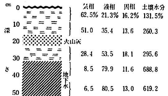
第3図 土壌相の垂直分布
