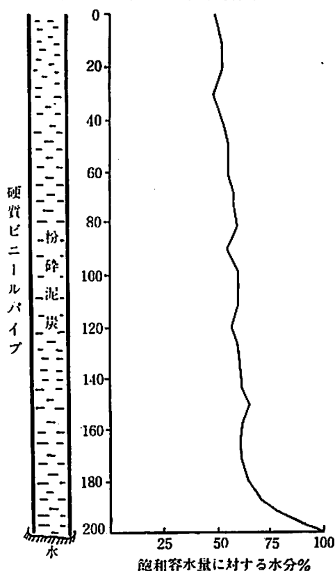
第4図 泥炭の垂直水分分布
