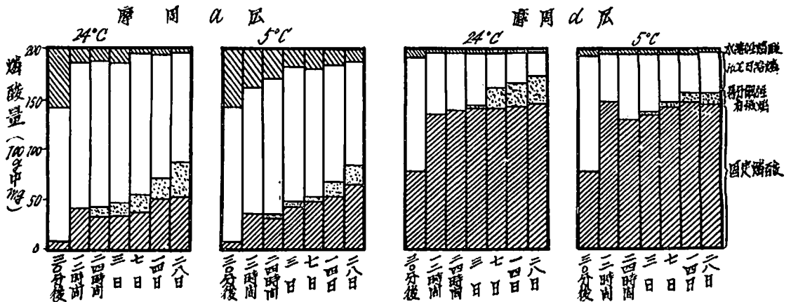
第 2 図 火山灰に \text{H}_3\text{PO}_4 を添加せる場合の有機燐生成経過
