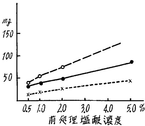
第3図 前処理塩酸濃度に対応する Simon 法 (N/8-NaF) \text{KMnO}_4 消費量 (a)
