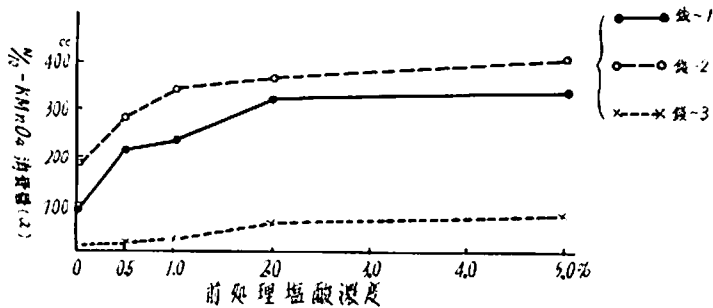
第3図 前処理塩酸濃度に対応する Simon 法 (N/8-NaF) \text{KMnO}_4 消費量 (a)
