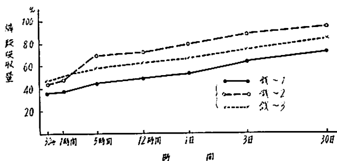
第8図 磷酸吸収量と時間
