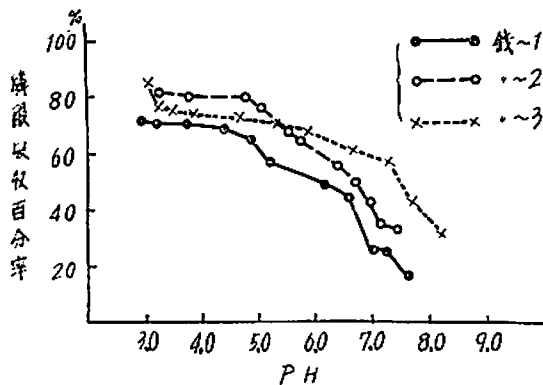
第7図 塩土の磷酸吸収型
