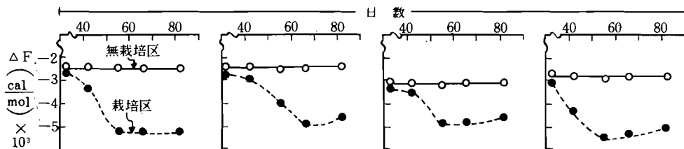
図4 供試土壌の加里置換エネルギーの推移
