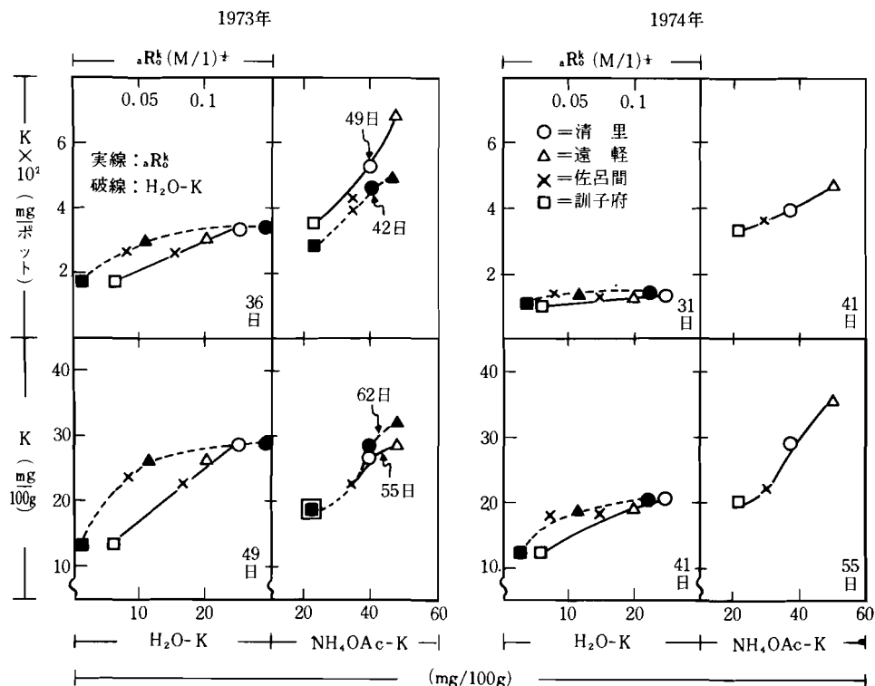
図 6 えん麦の加里吸収量と土壌中の H_2O-K 、 NH_4OAc-K 、 aR_b^k の関係
