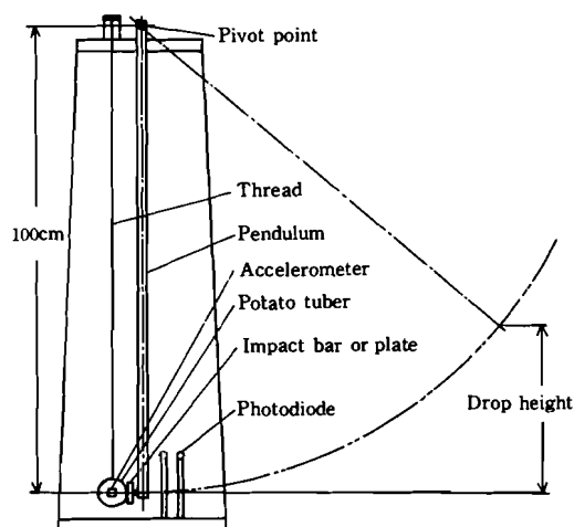
Fig. 1 Pendulum impact apparatus
