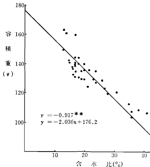
図3 U_0 — b_1 土壌の含水比と容積重の関係
