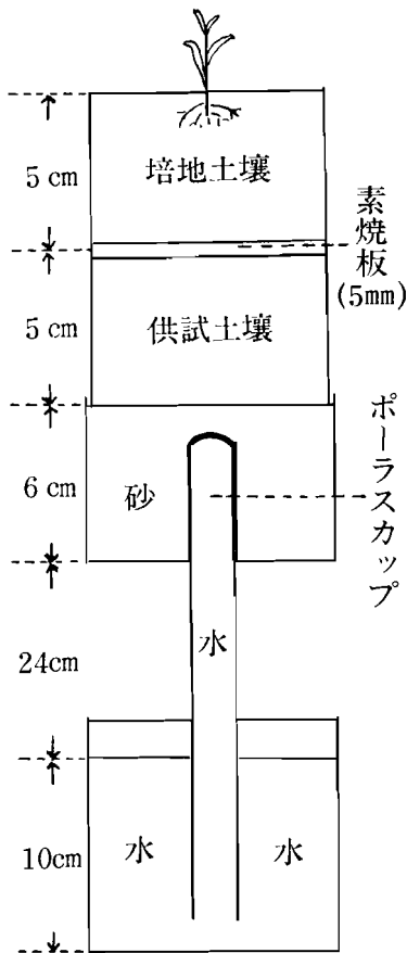
図 4 実験装置
