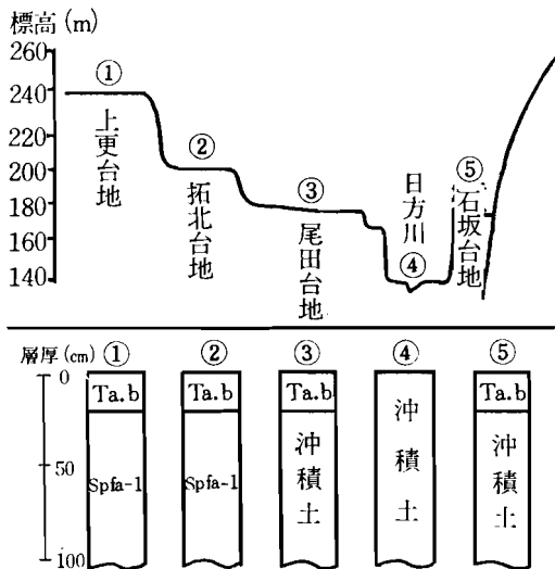
図 10 火山灰と地形面の堆積関係 (南部)
