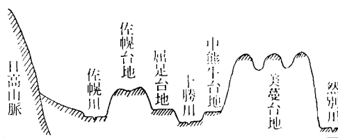
図4 西部の地形模式図
