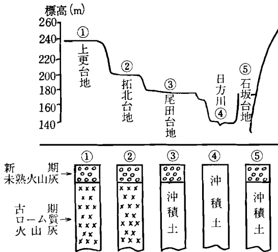
図 16 区分した火山灰の堆積関係 (南部)
