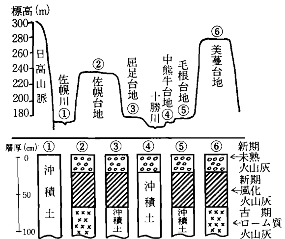
図 15 区分した火山灰の堆積関係 (西部)
