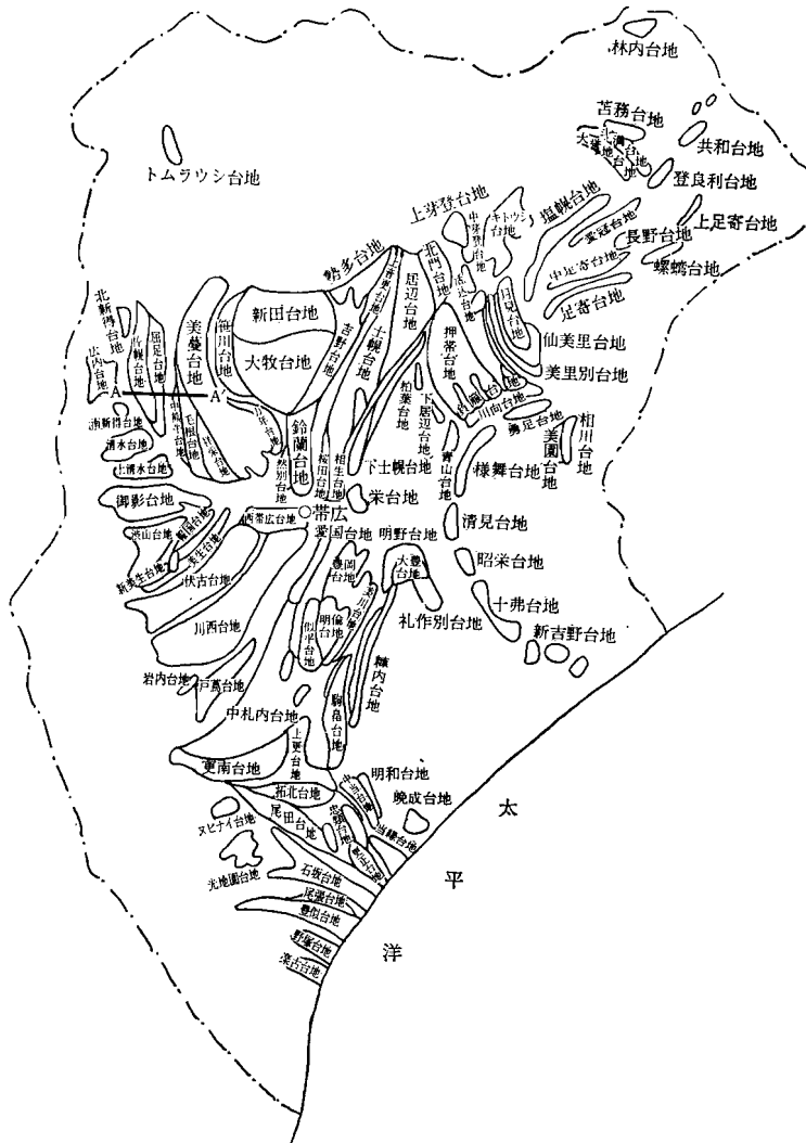
図1 十勝管内の台地区分図
