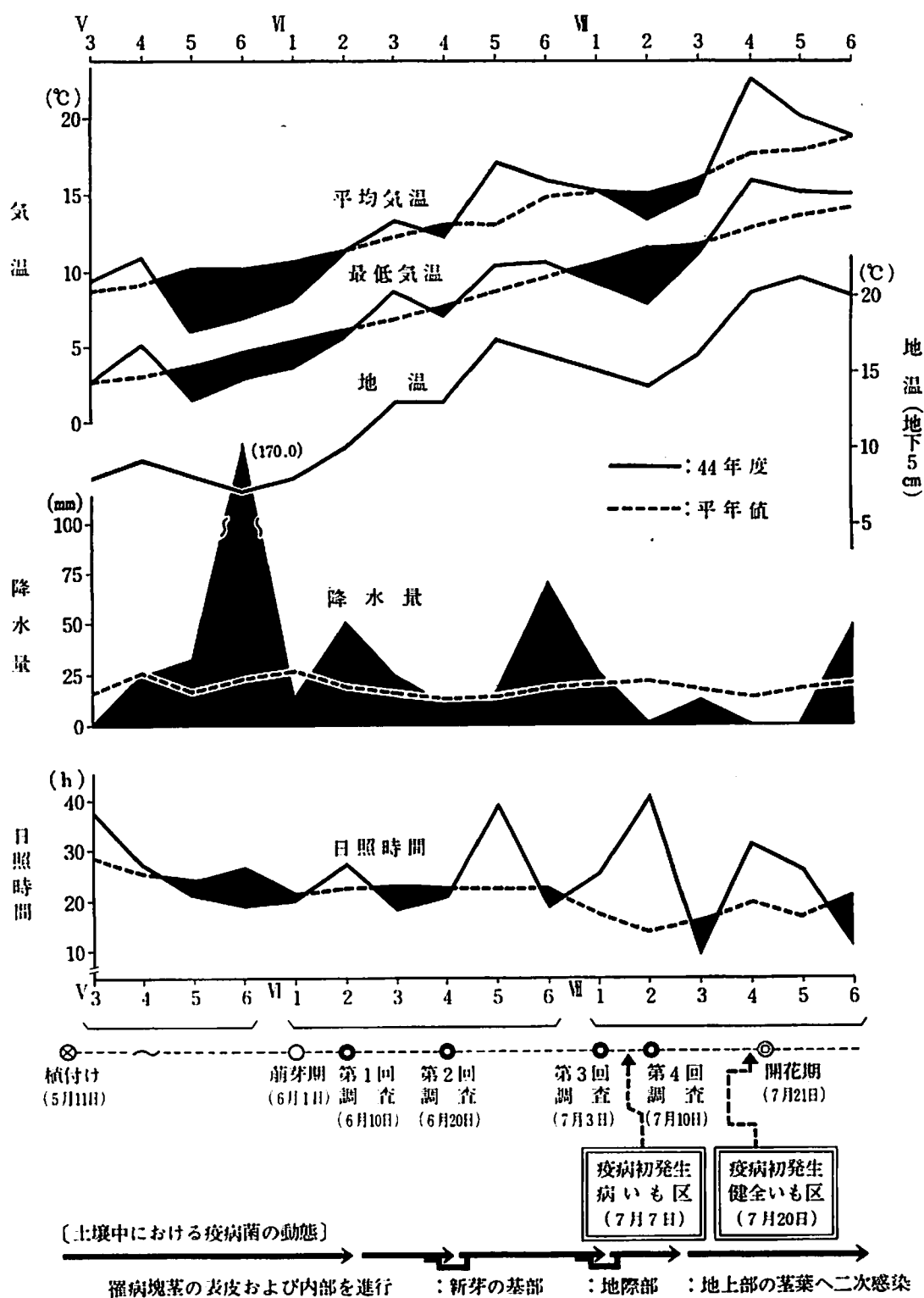
第4図 ほ場におけるばれいしょ疫病菌の生態と気象経過(半月別)との関係
