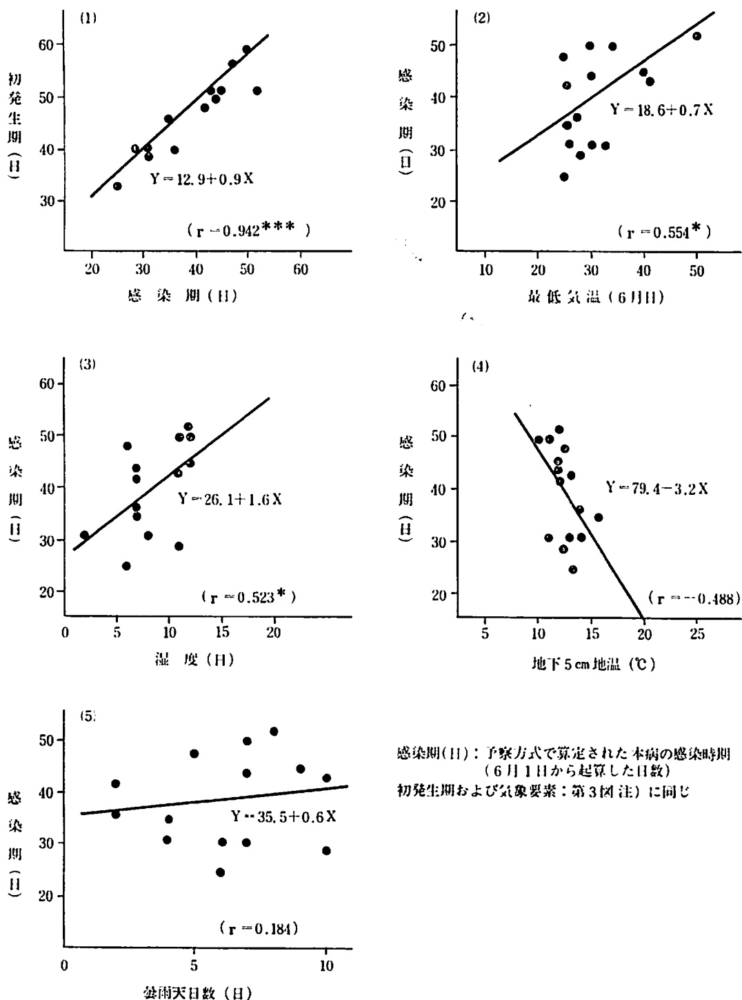
第5図 ばれいしと疫病の初発生期と感染期ならびに気象要素との関係
