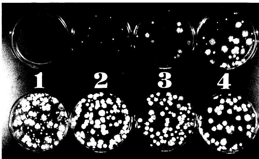
図版 1 太陽熱処理後の土層別糸状菌数 (村重 1986, ローズベンガル培地) 上段: 処理区 (マルチ+トンネル), 下段: 無処理区 土層番号 1: 0~5 cm, 2: 5~10cm, 3: 10~15cm, 4: 15~20cm
