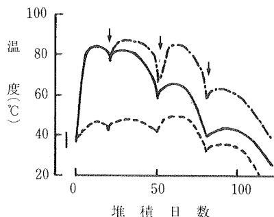
図3 堆積過程の温度変化に及ぼす添加物の影響 ——鶏糞+尿素 ——全量鶏糞 -----全量尿素 矢印は切り返しを示す。
