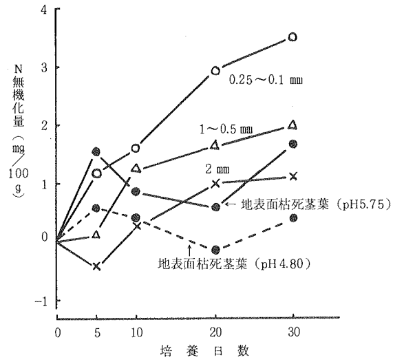
図1. 各粒径別有機物のN無機化量 培養条件：乾土10g当り有機物-C 50mgおよび硫酸-N 2mg添加，ほ場含水量で培養，有機物無添加区との差からN無機化量を算出した。
