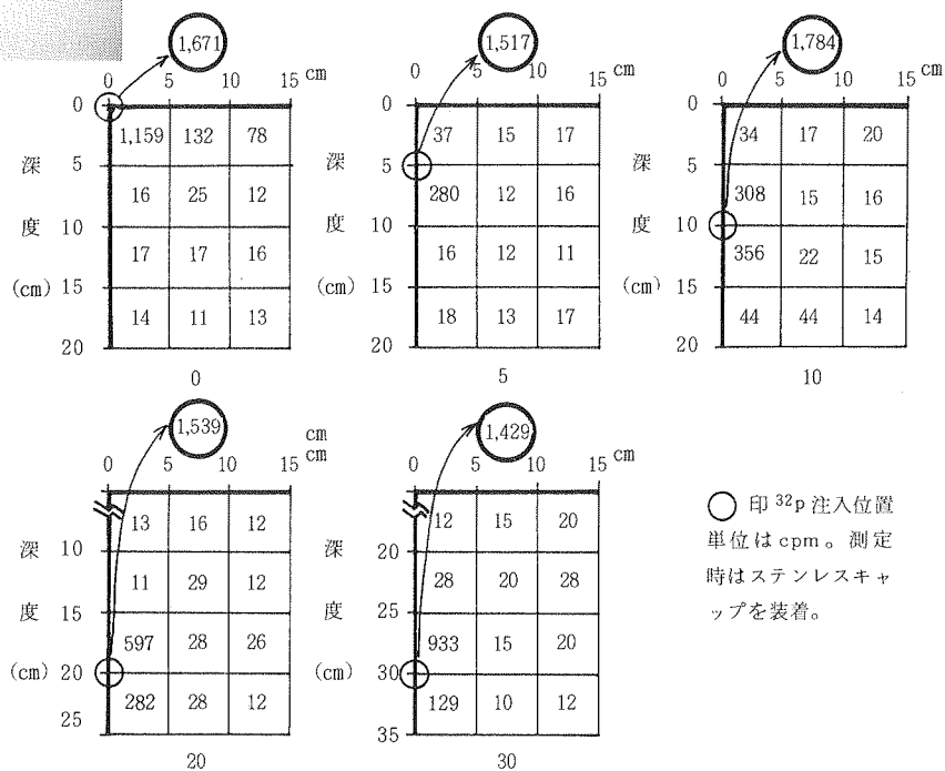
図3. 土層内における ^{32}\text{P} の分布
