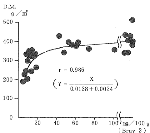
図 6. 土壌りん酸含量と牧草乾物収量
