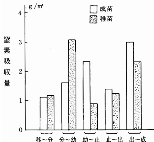
第3図 生育時期別の窒素吸収増加量
