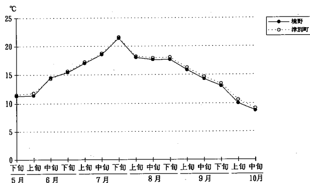
図1 津別町と境野における平均気温の推移 (1995～1997年)
