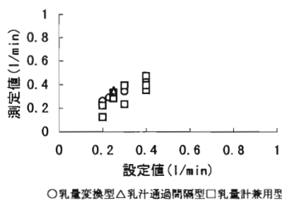
図3 離脱作動時の流量 (電気伝導度, ハイライン)
