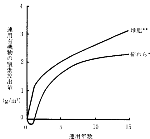
図5 稲わら・堆肥連用時の窒素放出の推移(計算値)
