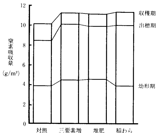
図1 生育時期別窒素吸収量 (10カ年平均)
