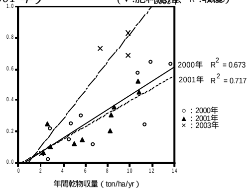
図3 乾物収量と亜酸化窒素発生量との関係 (2000,2001,2003 年)
