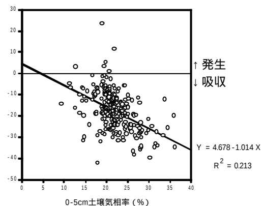
図6 表層0 ~5cm 土壌気相率とメタン発生フラックスの関係 (2000 ~2003 年)
