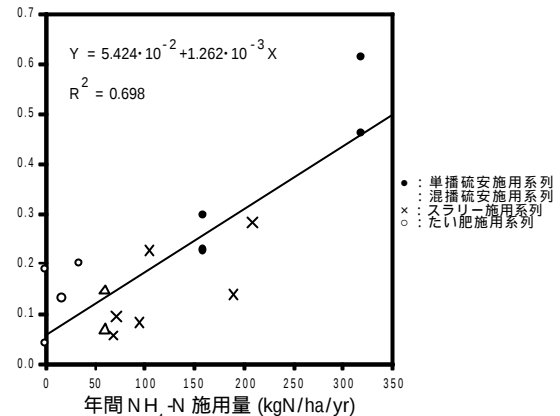
図2 年間アンモニア態窒素施用量と施肥由来 亜酸化窒素発生量の関係 (2000 ~2001 年)
