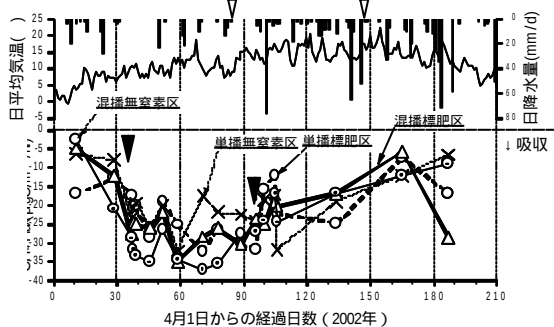
図5 採草地におけるメタン発生フラックスの推移 (2002 年) (:肥料施用, :収穫)
