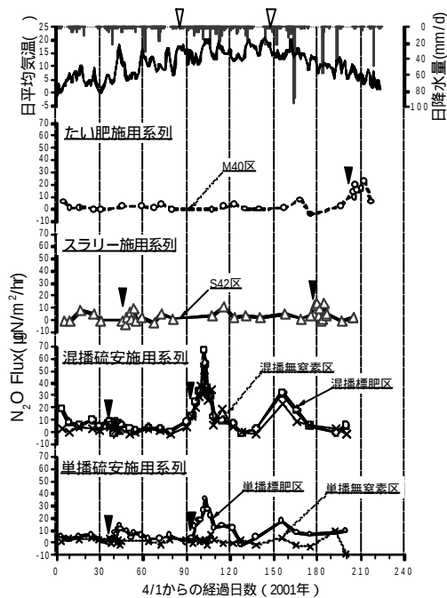
図1 亜酸化窒素発生フラックスの推移 (2001 年) (▼:肥料施用, R²:収穫)
