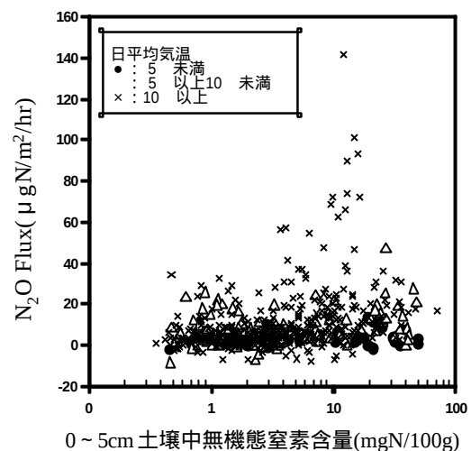
図4 平均気温別土壤中無機態窒素含量と亜酸化窒素発生フラックスの関係 (2000 ~2001 年)
