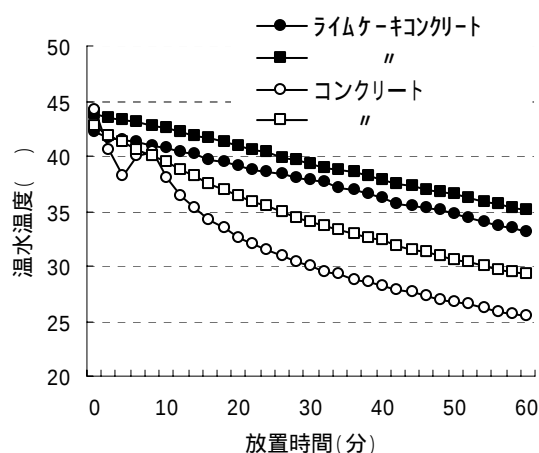
図1 ライムケーキコンクリート舗装またはコンクリート舗装に放置した温水の温度変化 (ビニール袋に5Lの温水(43℃)を入れ、各パドック上に放置。気温:7℃)
